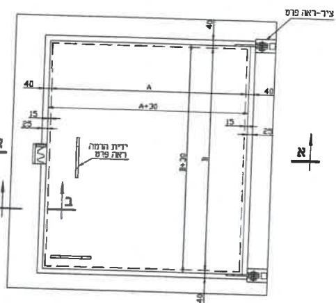
תוכנית המכסה
