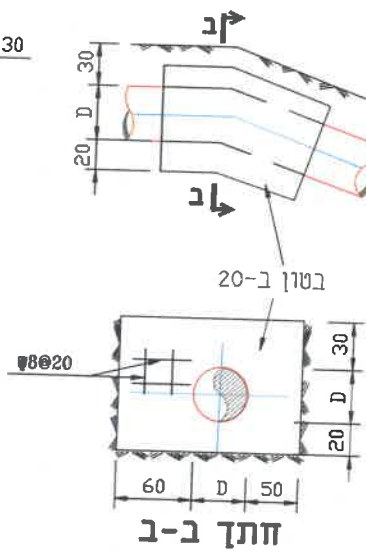
פרט D
