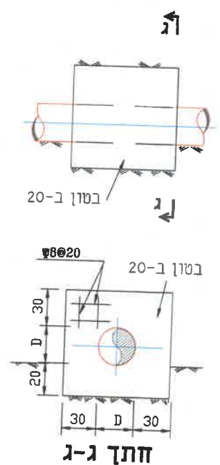
פרט E
